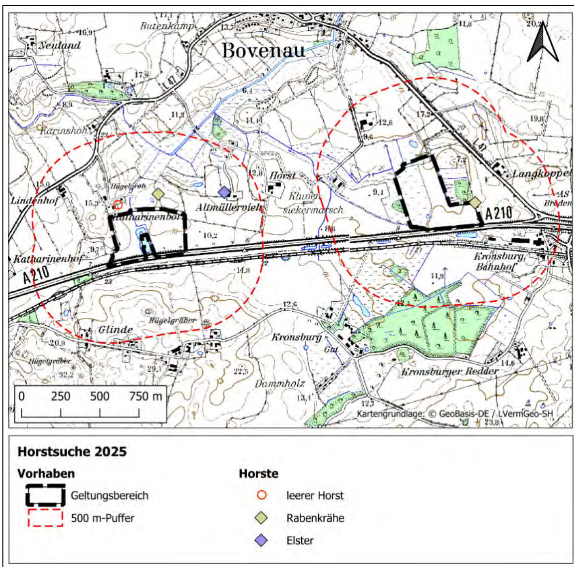
Abb. 16: Ergebniskarte Horstsuche
